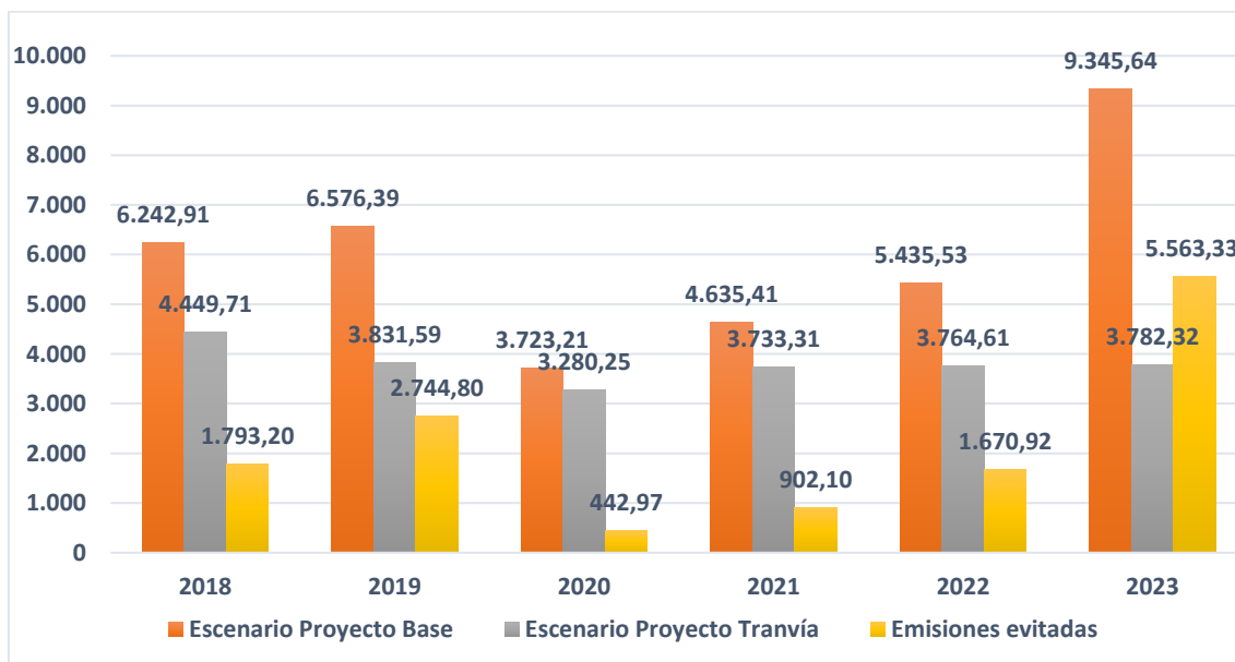
Figura 6. Evolución de las emisiones de GEI en cada escenario y estimación de las emisiones evitadas (tCO 2 e)
